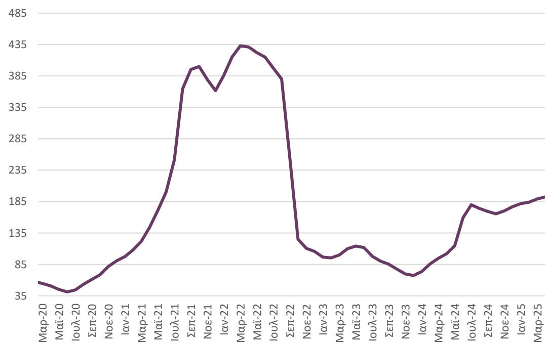
Δείκτης εμπορευματοκιβωτίων (1999=100)
